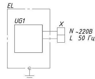
Рисунок 2 – Электрическая схема подключения
