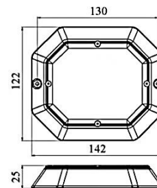
Рисунок 1 – Габаритные размеры светильника
